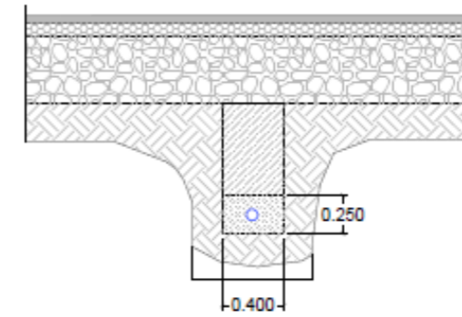
Sezione tipo B-B
