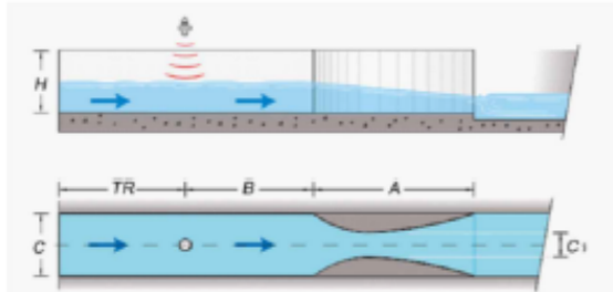
STANDARDIZZAZIONE DEL CANALE IN BASE ALLA PORTATA
