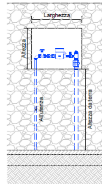
Prospetto
