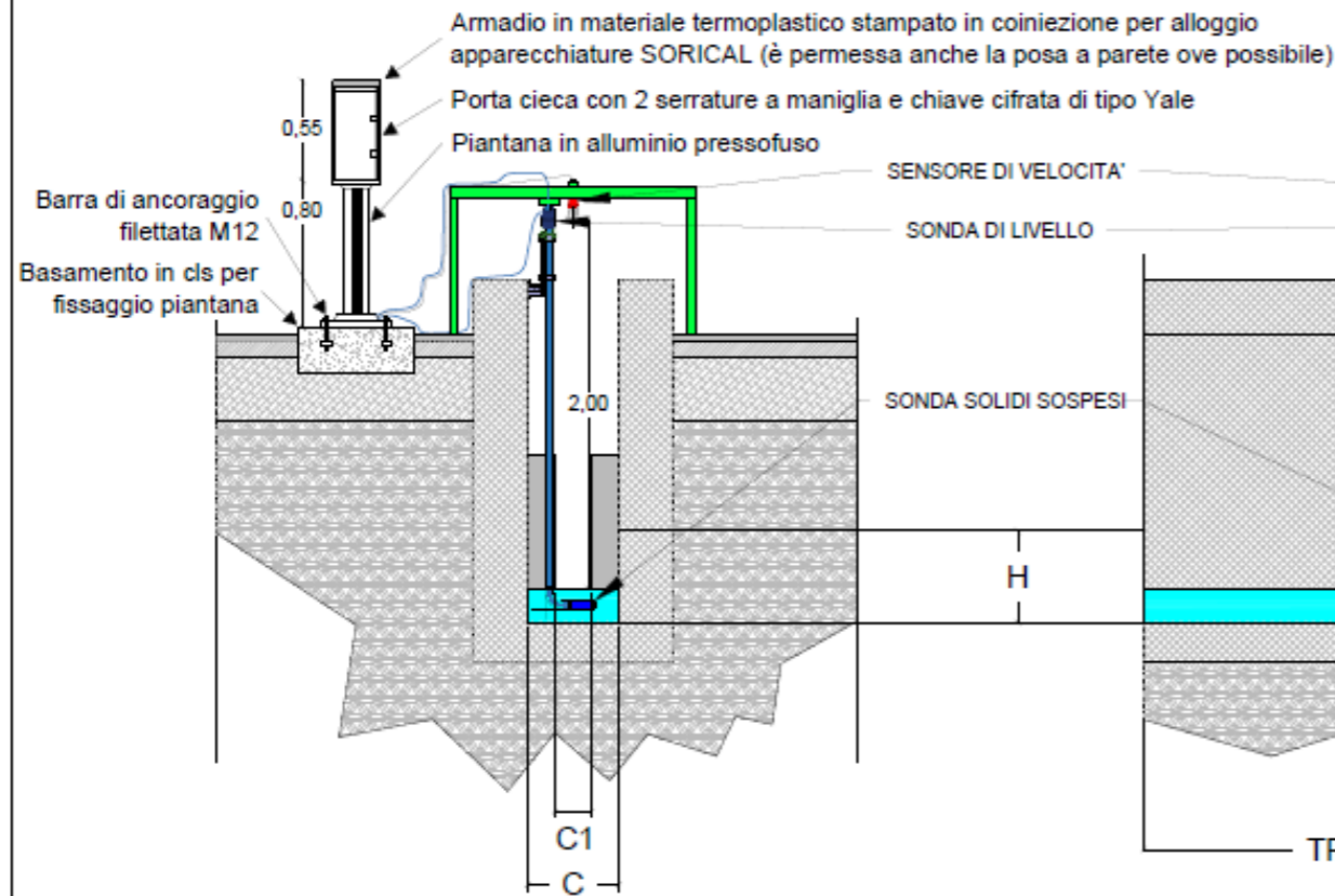
Sezione B-B
