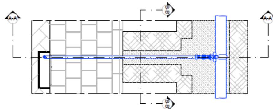
Derivazioni allacci privati con collare di presa
