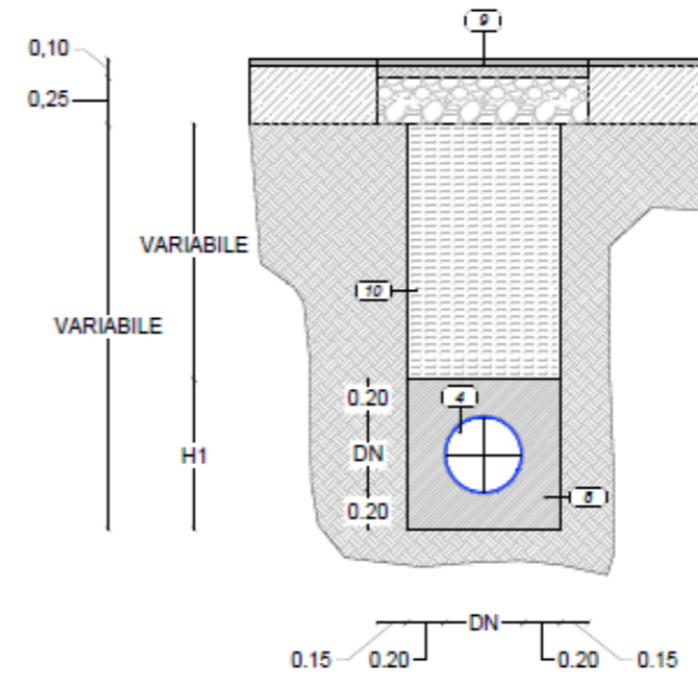
Sezione tipo B-B
