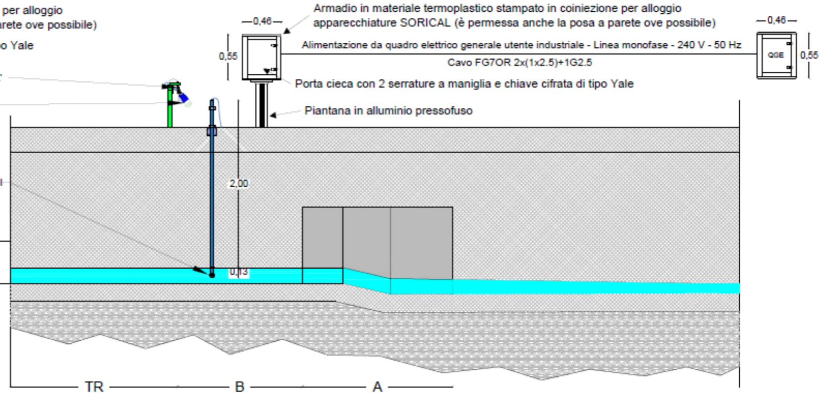
Sezione A-A
